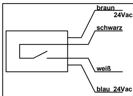
elektrischer Anschluß
