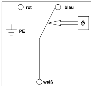
Anschlußschaltbild
