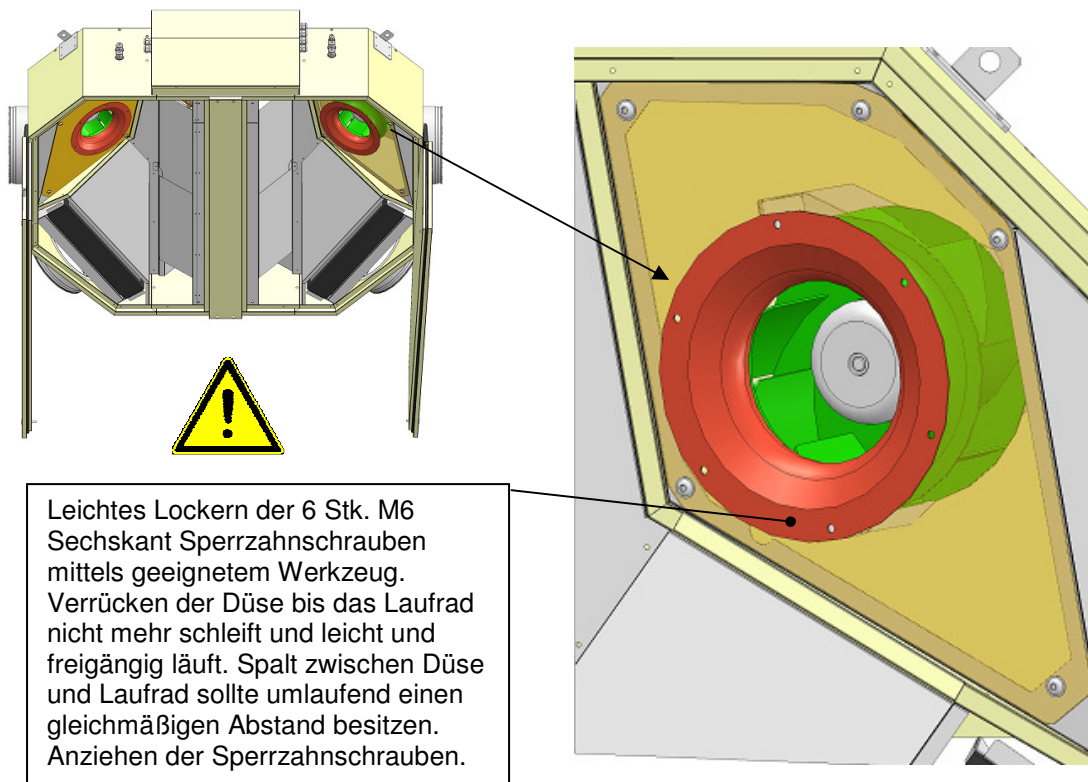
Abbildung.: Justieren der Düse
