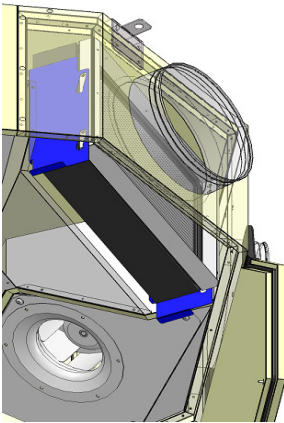
Abbildung: Panelfilter Deckengerät
