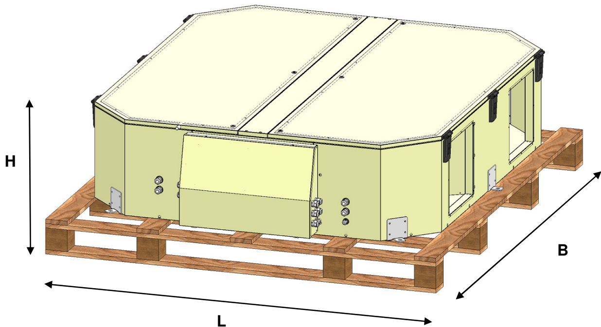
Abbildung: Transportmaße SupraBox 1900D
