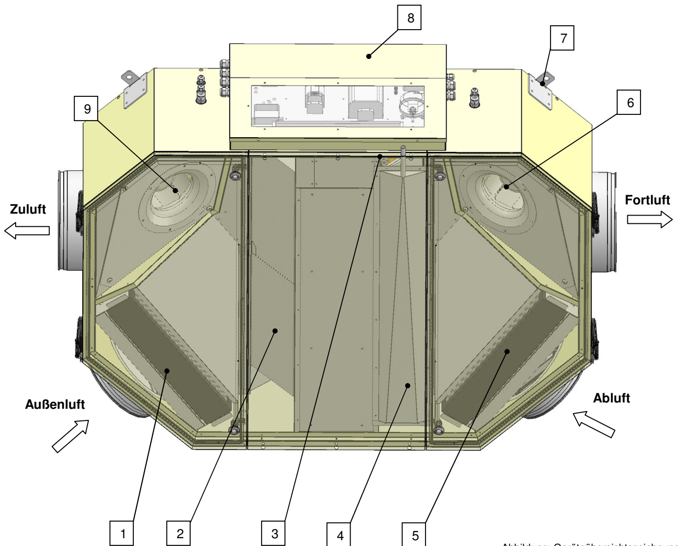
Abbildung: Geräteübersichtszeichnung SBC110DGRIB0
